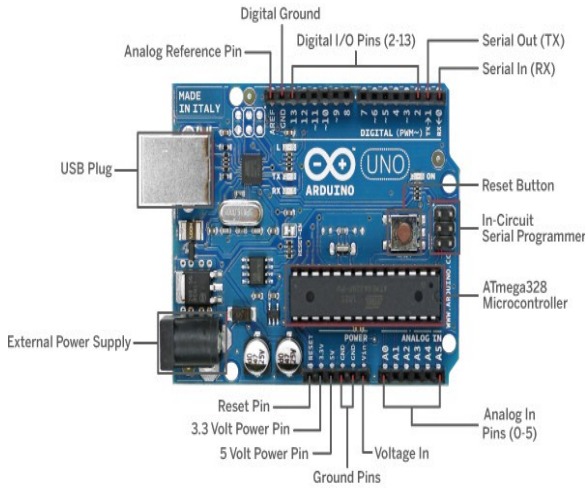
Fig. 3. Arduino UNO R3
