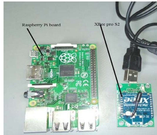
Fig. 8. WSN node
