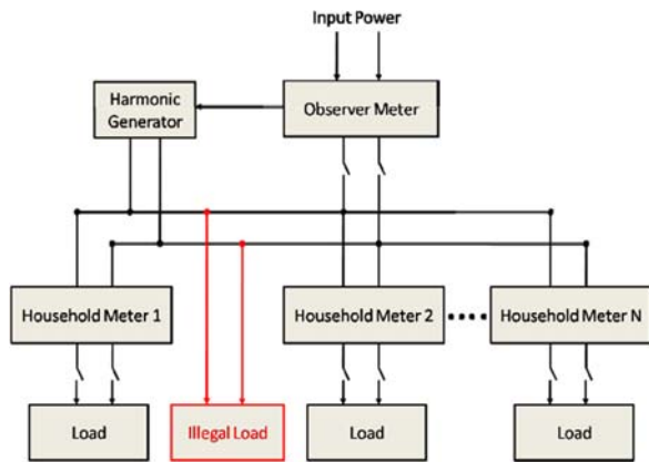
Fig: 8 : Unregistered load or Illegal load
