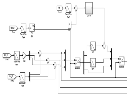
Fig. 6.6: Reference dq component generation using DSM-PI controller
