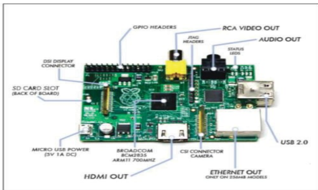
Fig. 3. Raspberry pi-3
